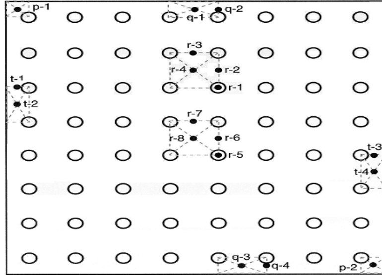
Figura 490.1 a. Puntos de medición de iluminancia en la cuadrícula de un local con luminarias espaciadas simétricamente en dos o más filas
