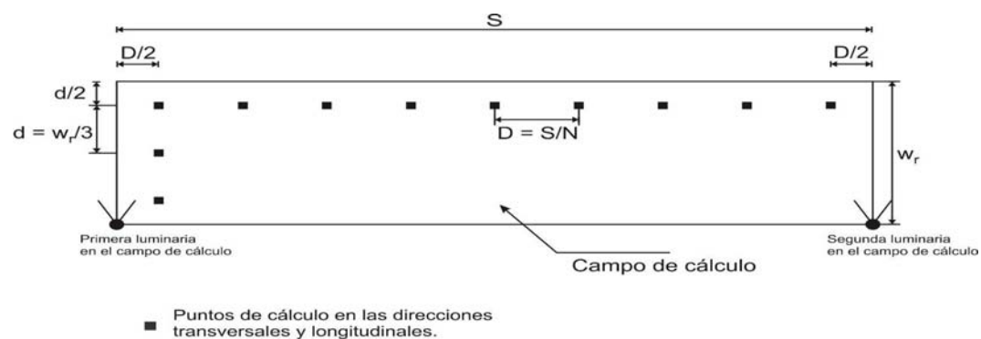
Figura 530.3.1. Puntos de cálculo para la iluminación
