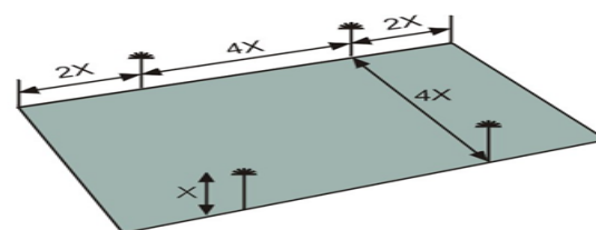
Figura 560.1 b. Ubicación de mástiles laterales al área
