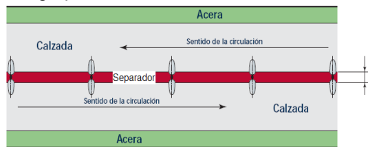
Figura 510.5.1 b. Disposición Central doble (para 1,5 \text{ m} \geq b \leq 4 \text{ m} )
